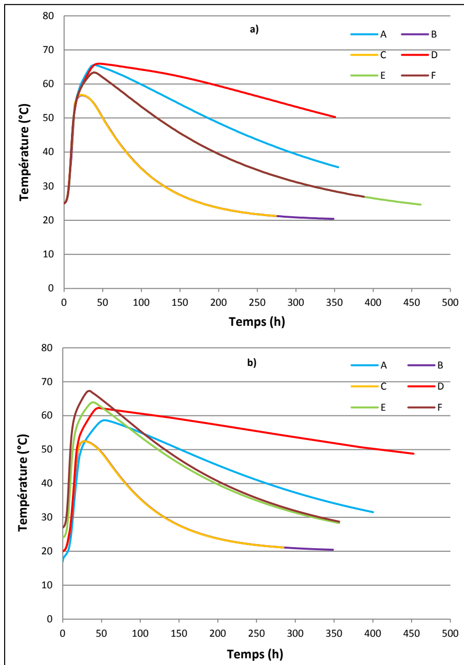
Figure II.4 : évolution des températures maximales dans les différents plots du radier : cas du calcul en prenant une température identique de bétons frais égale à 25°C (a), cas du calcul en tenant compte de la différence des températures réellement mesurées dans les bétons frais (b) (Tableau II.2)
